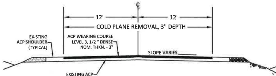
KNOTT RD STA. 145+00 - STA. 215+00
