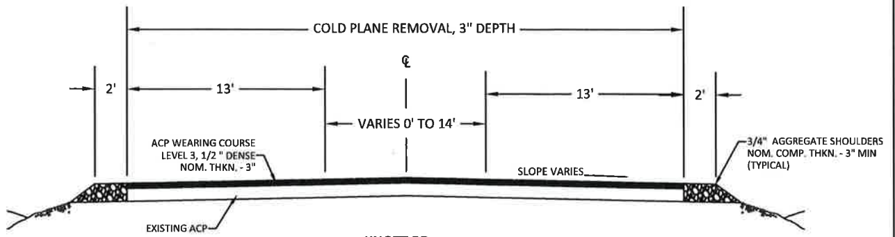
KNOTT RD STA. 0+00 - STA. 4+50 STA. 61+00 - STA. 68+02
