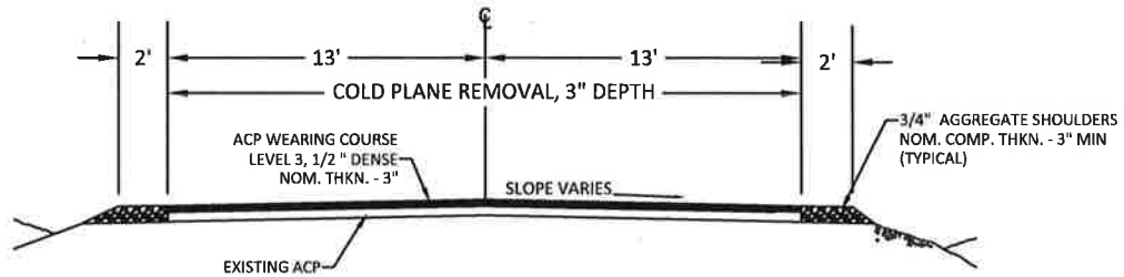
KNOTT RD STA. 4+50 - STA. 61+00
